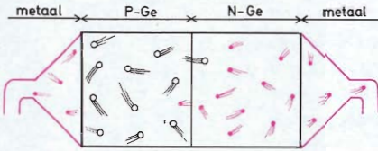
Fig. 15. Grensverkeer van de vrije elektronen en gaten
