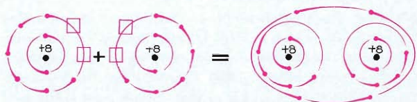
Fig. 7. Twee zuurstofatomen geven een zuurstofmolecuul
