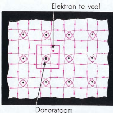
Fig. 13. N -germanium
