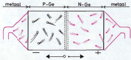
Fig. 16. Het overgangsgebied bij de grens tussen P- en N-germanium
