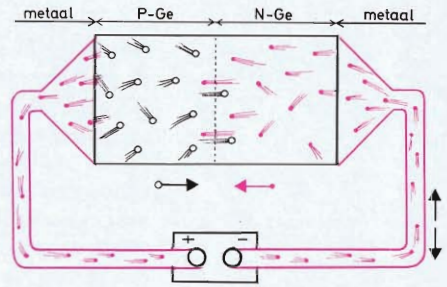
Fig. 18. Diode geschakeld in doorlaatrichting
