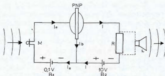
Fig. 23. Schakeling van een transistor als versterker
