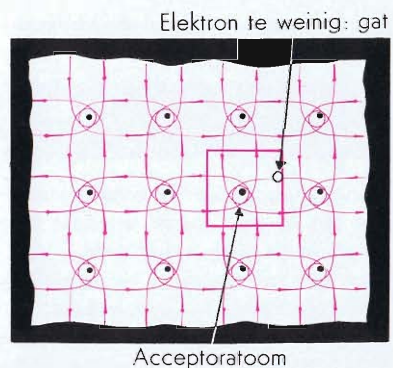
Fig. 14. P -germanium
